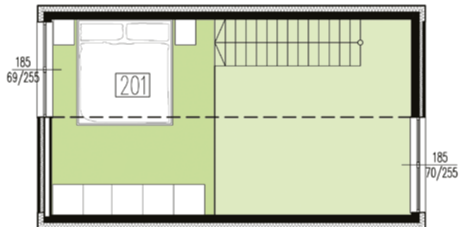
RZUT ANTRESOLI
