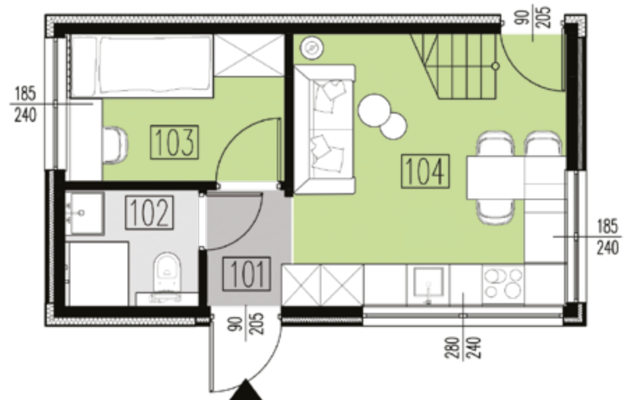
RZUT PARTERU
