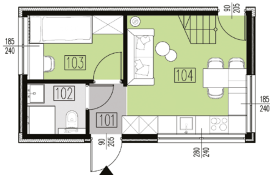
RZUT PARTERU
